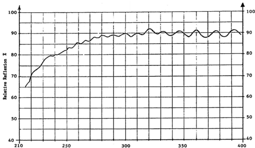
Reflexion in Abhängigkeit von der Wellenlänge
